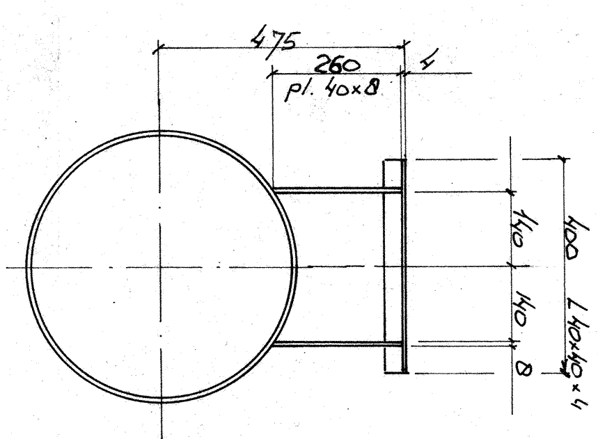
Doorsnede C-C
